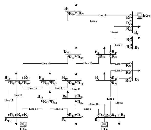
شکل (۳): نمایش تک خطی بخش توزیع شبکه ۳۰ شین IEEE
