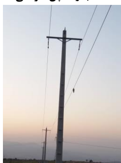
شکل ۱۵: عدم استحکام مناسب سرتیری مهره‌خور سیلیکونی استفاده شده
