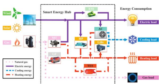
شکل ۲: یک نمونه هاب انرژی با مصارف متعدد (Wang, Zhong, Ma, Xia, & Kang, 2017)
