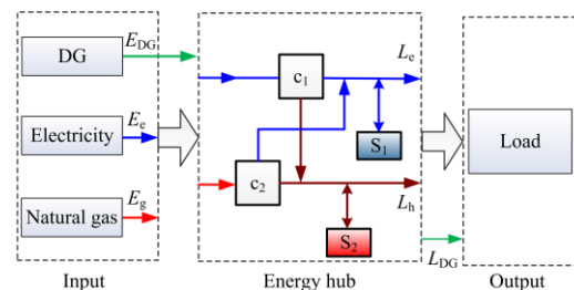
شکل ۵: مدل‌سازی ورودی و خروجی هاب انرژی (Ha et al., 2017)
