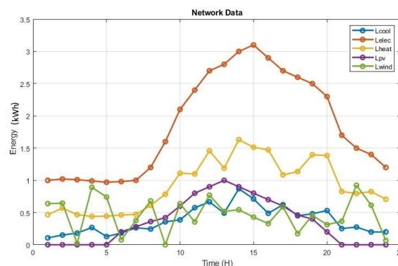
شکل ۱۰: داده‌های بارهای شبکه (de Jong, Sánchez, Esquerre, Kalid, & Torres, 2013)
