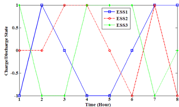
شکل ۶: دیگرام الگوی شارژ-دشارژ باتری ها
