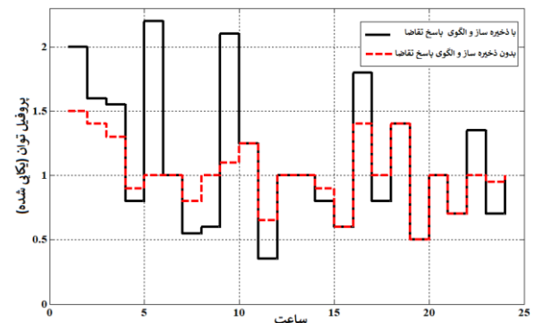
شکل ۱۰: پروفیل توان با و بدون اعمال روش پیشنهادی
