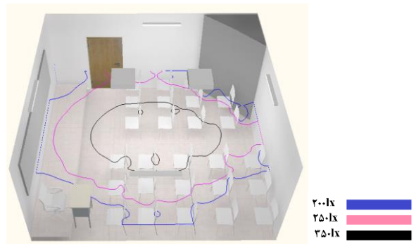
شکل (۳): شبیه سازی کلاس ۲۰۶ در نرم افزار دیالوکس
