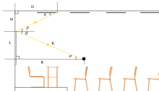
شکل (۵): حداکثر فاصله ی لامپهای ردیف اول از تخته
