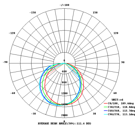
شکل (۱): منحنی پخش نور پنل LED ۶۰×۶۰ [۱۹]
