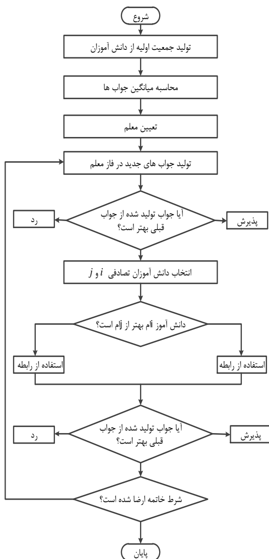
شکل ۱: فلوچارت الگوریتم TLBO
