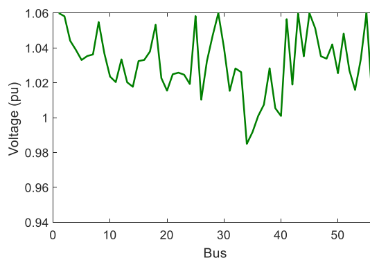
شکل ۹: پروفیل ولتاژ تمامی باس‌ها
