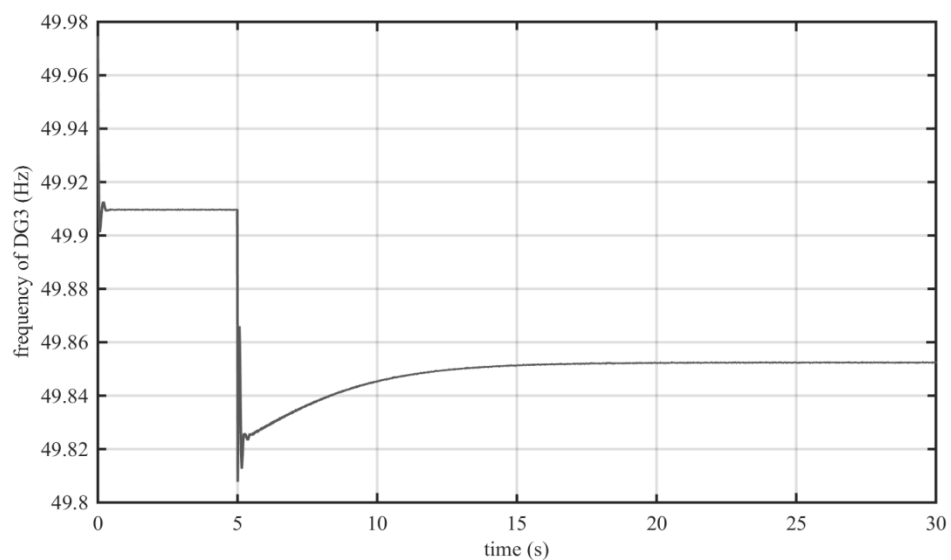
شکل (۸): فرکانس منابع تولید پراکنده در ریزشبکه با کنترل کننده پیشنهادی تخصیص توان در شرایط تغییر آنی بار و با حضور منبع دارای دینامیک در تولید انرژی
