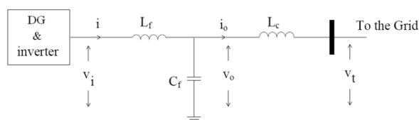
شکل (۱): منبع تولید پراکنده متصل به شبکه
