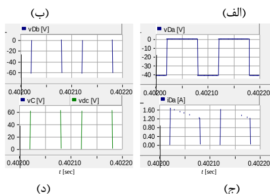
شکل ۱۸- شکل موج‌های ولتاژ و جریان اجزای S-ZSI با استفاده از روش کلیدزنی PWM مدولاسیون سینوسی؛ (الف) ولتاژ و جریان عبوری از سلف L ؛ (ب) ولتاژ و جریان عبوری از
