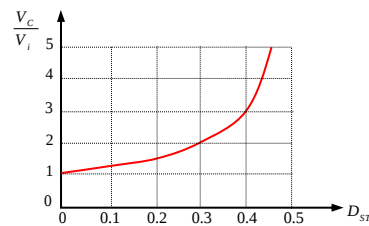
شکل ۵- مشخصه انتقال S-ZSI
