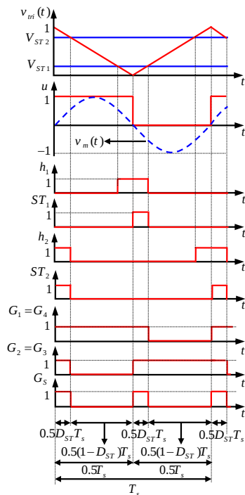
شکل ۱۱- تولید سیگنال‌های ST در یک دوره تناوب برای
