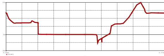
شکل (۷) شکل موج جریان سوئیچ M_1 (1 μs/div, 4 A/div)
