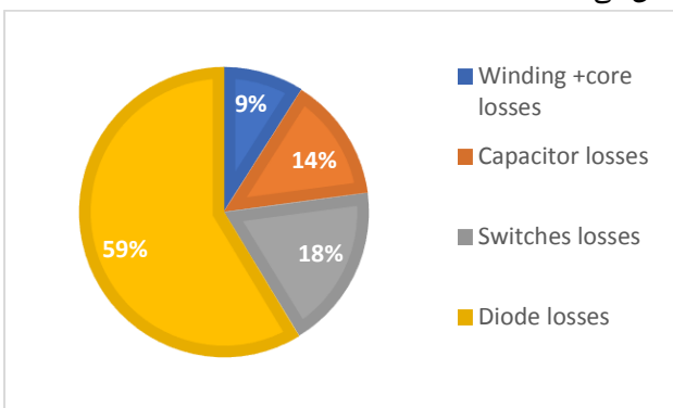
شکل (۱۵) نمودار توزیع تلفات المانهای مبدل پیشنهادی
