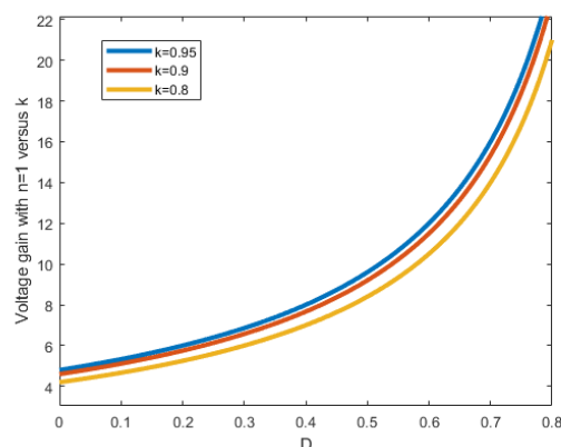
شکل (۵): نمودار بهره مبدل بر حسب تغییرات ضریب تزویج
