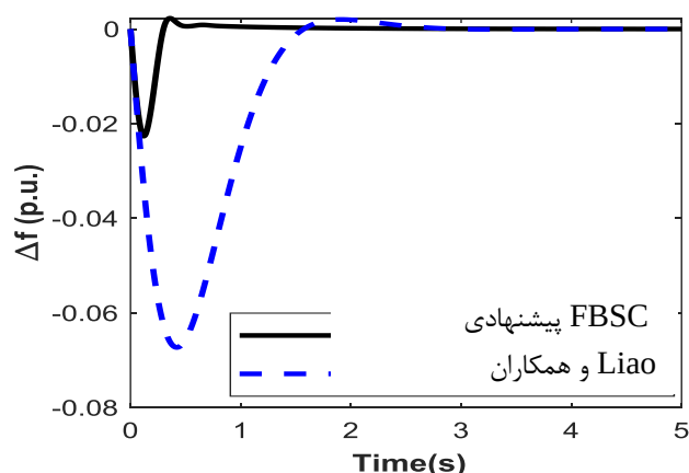
شکل ۴: پاسخ دینامیکی تغییرات فرکانسی سیستم
