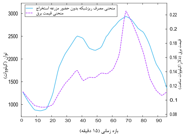
شکل (۲): منحنی تقاضا و قیمت برق ریزشبه
