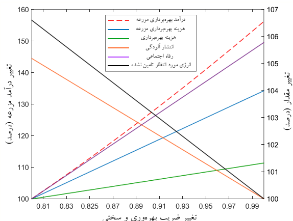
شکل (۹): آنالیز حساسیت نسبت به تغییرات ضریب بهره‌وری و سختی.
