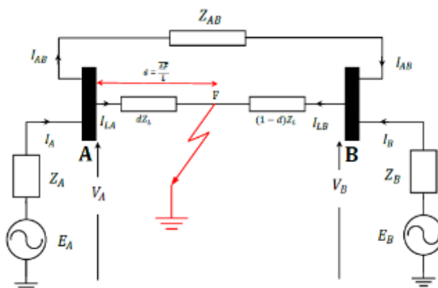
شکل (۳): وقوع خطا اتصال کوتاه تک فاز به زمین در خط AB
