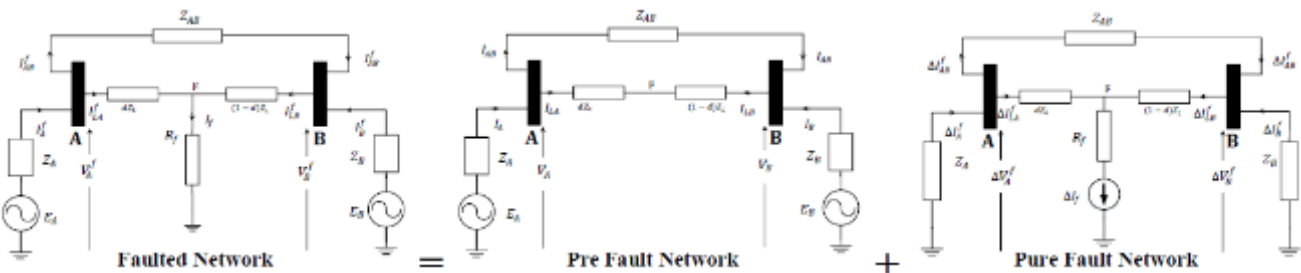
شکل (۵): تفکیک شبکه‌ی خط‌آلود به شبکه‌ی قبل از خطا و شبکه‌ی تحت جریان خطای خالص
