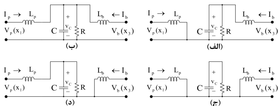
شکل (۲): مدهای کاری مدار سوئیچینگ، الف: (SW1 بسته، SW2 بسته و SW3 باز)، ب: (SW1 بسته، SW2 باز و SW3 بسته)، ج: (SW1 باز، SW2 بسته و SW3 باز)، د: (SW1 باز، SW2 باز و SW3 بسته)
