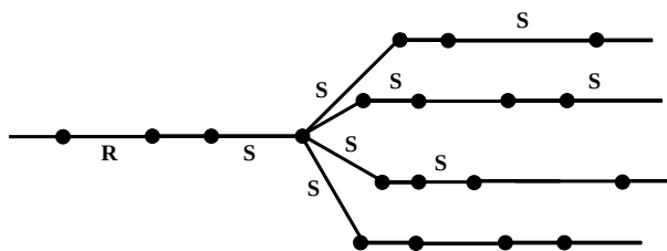
شکل ۲. برقراری شرط حداکثر سکشن لایزهای تحت یک ریکلوز
