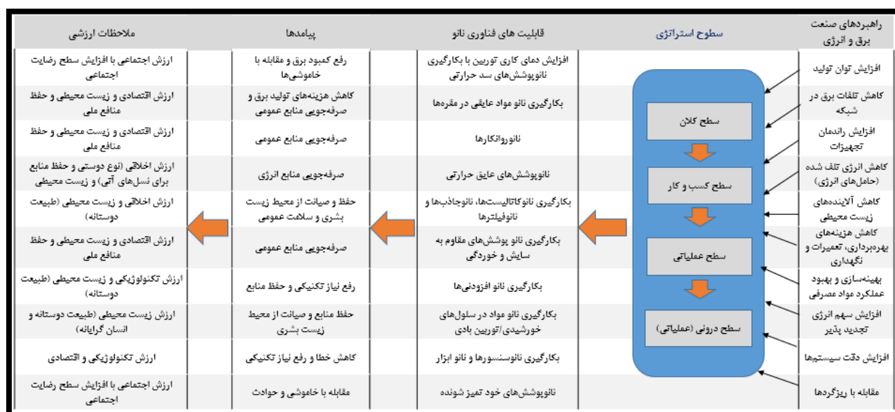
شکل (۶) سنجش قابلیت‌های فناوری نانو در راستای راهبردهای صنعت برق و انرژی با تأکید بر ضرورت ملاحظات ارزشی (نتیجه تحقیق)
