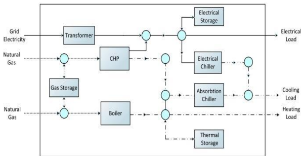
شکل ۱: ساختار کامل یک هاب انرژی
