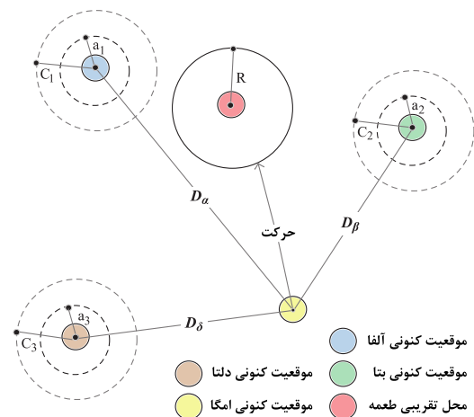
شکل ۷: موقعیت شکار و شکارچی در الگوریتم گرگ خاکستری (Rodríguez, Castillo, & Soria, 2017)
