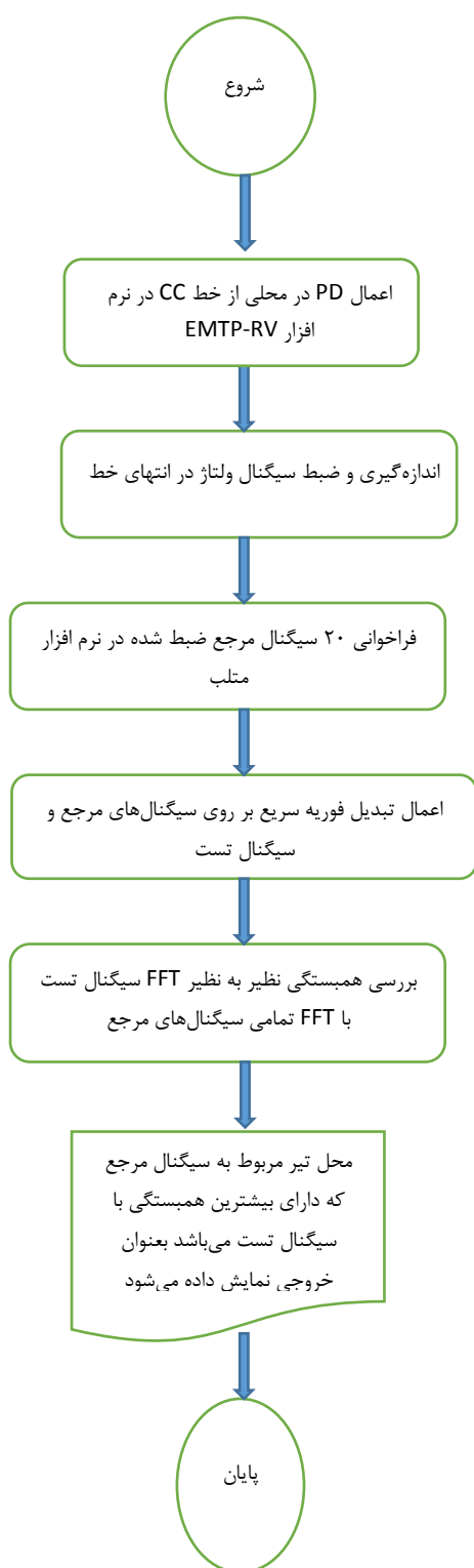
شکل (۵): الگوریتم روش پیشنهادی جهت تشخیص محل وقوع تخلیه جزئی
