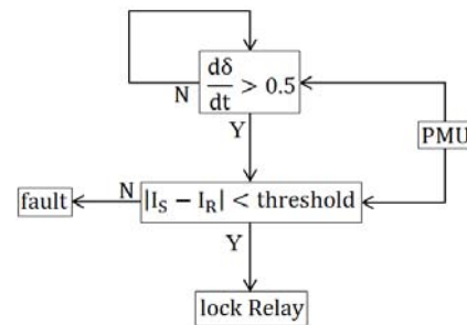
شکل (۲): فلوچارت روش جریان محور
