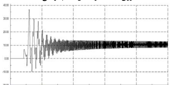
شکل (۵) زاویه شین B1 در شبکه ۱۴ شینه در صورت وقوع خطا روی خط L7 و اعمال نشدن اقدام درمانی
