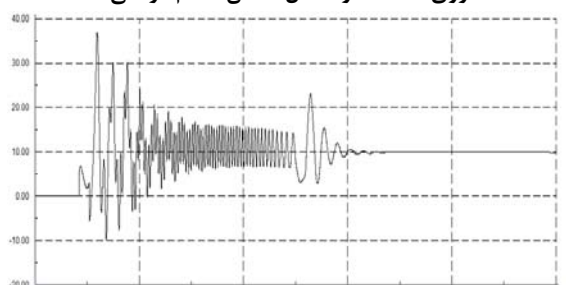
شکل (۶) زاویه شین B1 در شبکه ۱۴ شینه در صورت وقوع خطا روی خط L7 و اعمال اقدام درمانی
