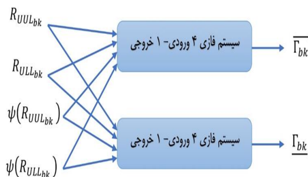
شکل ۲: ساختار الگوریتم انفیس
