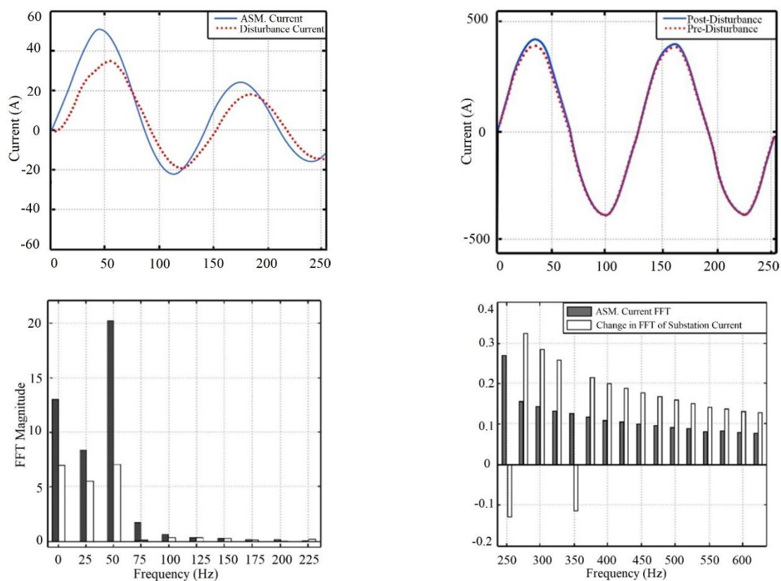
شکل (۹): وصل موتور القائی (موتور ۲۵۰ کیلووات ۶ کیلوولت متصل به گره ۴۰)
