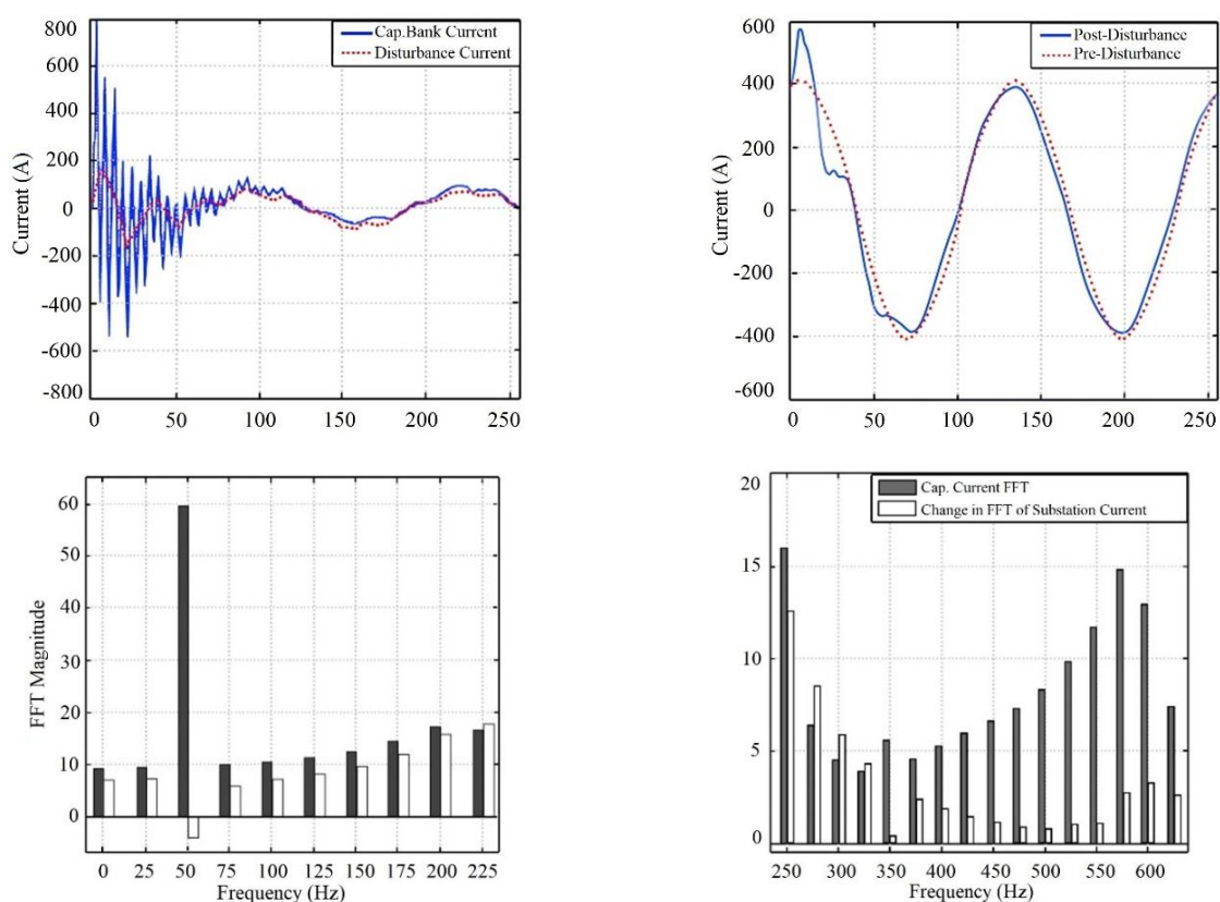
شکل (۸): وصل بانک خازنی (بانک خازنی متصل به گره ۲۴)
