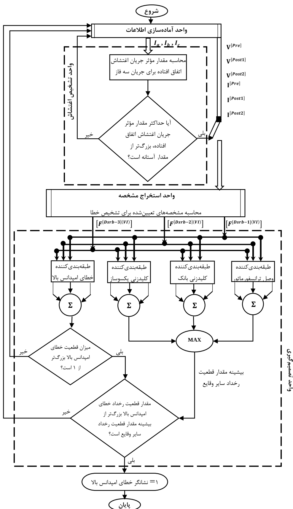
شکل (۲): روند نمای کلی تشخیص خطای امپدانس بالا
