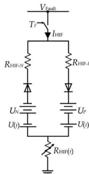
شکل (۴): مدل مداری خطای امپدانس بالای شبیه‌سازی‌شده
