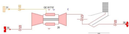
شکل ۴- سیکل ساده توربین گاز بدون خنک‌کاری
