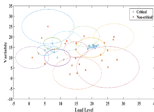
شکل (۳): دسته‌بندی ۴۶ نقطه کار با استفاده از الگوریتم تابع پایه‌ای شعاعی
