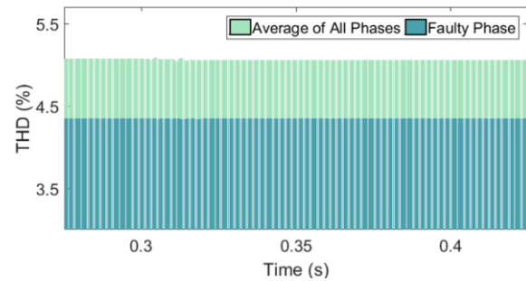
شکل (۱۲): عملکرد روش مبتنی بر THD جریان هنگام وقوع خطای امپدانس بالا در باس ۶۳۲ در حضور بار غیرخطی
