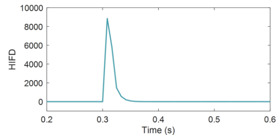
شکل (۱۰): شاخص پیشنهادی هنگام کلیدزنی بار در باس ۶۷۱
