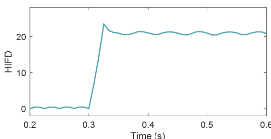
شکل (۹): شاخص پیشنهادی هنگام وقوع خطا در باس ۶۵۲
