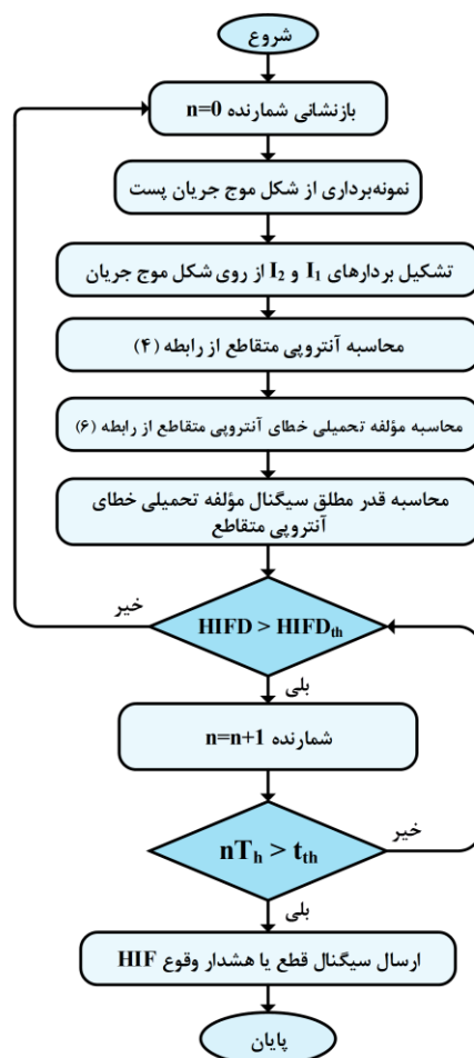
شکل (۷): روندنمای الگوریتم آشکارسازی خطای امپدانس بالای پیشنهادی
