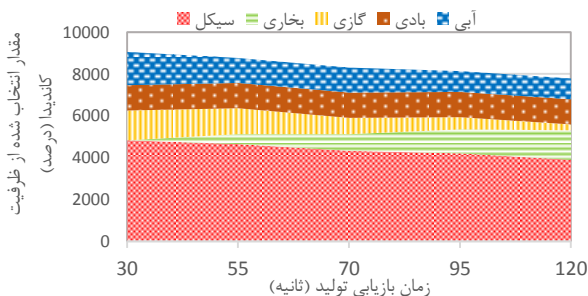
شکل (۵): ظرفیت بهینه‌ی نیروگاه‌ها برای مقادیر مختلف زمان بازیابی تولید
