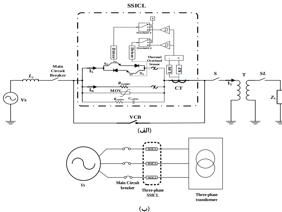
شکل (۱): الف) ساختار تکفاز SSICL پیشنهادی (ب) ساختار سه فاز
