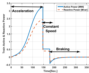
شکل (۶): نمودار توان اکتیو و راکتیو در نظر گرفته شده برای مدل بار قطار [18]
