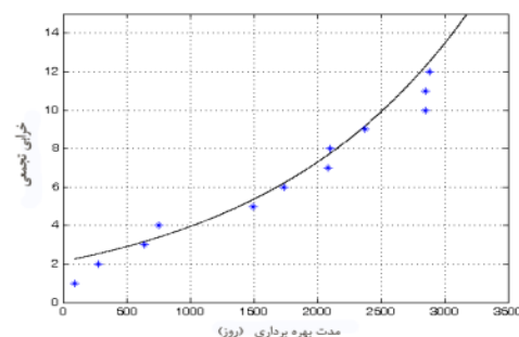
شکل (۷) تعداد تجمعی خرابی‌ها برحسب زمان‌های تجمعی و منحنی برازش شده برای فرآیند CP ترانسفورماتور
