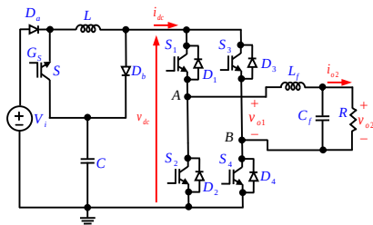
شکل ۲- ساختار S-ZSI
