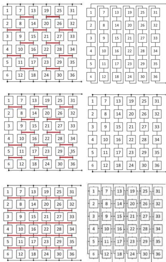
شکل (۷): پیکربندی‌های سری (بالا-راست)؛ سری-موازی (وسط-راست)؛ موازی (پایین-راست)؛ پل لینک دار (چپ-بالا)؛ شانه عسل (چپ-وسط)؛ پل کاملاً متقاطع (چپ-پایین).
