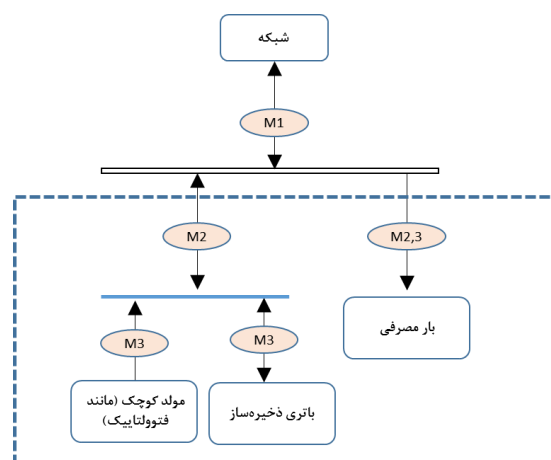
شکل ۳. آرایش‌های مختلف قرارگیری کنتور برای مشترکین کوچک
