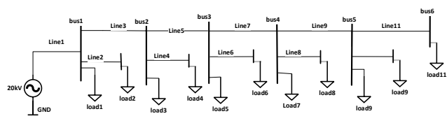
شکل (۲): نمودار تک خطی فیدر شبکه‌سازی شده
