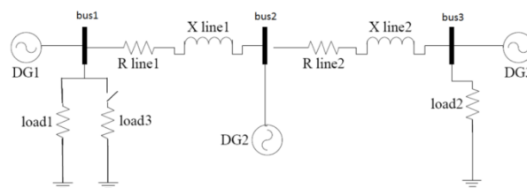
شکل (۵): ساختار ریزشبکه نمونه مورد آزمایش
