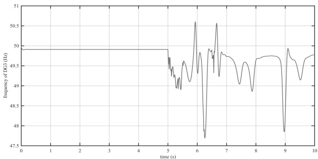
شکل (۷): ناپایداری فرکانسی سه منبع تولید پراکنده ریزشکه با کنترل کننده مرسوم تخصیص توان در شرایط تغییر آنی بار و با حضور منبع دارای دینامیک در تولید انرژی
