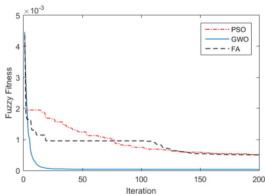
شکل (۲): نمودار همگرایی الگوریتم‌های PSO, GWO, FA و سناریوی اولیه
