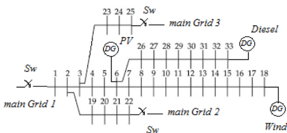
شکل (۱): شبکه تست نمونه ۳۳ باسه IEEE ریزشبهه
