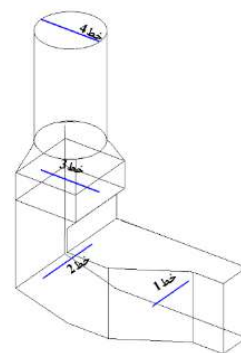
شکل ۵-۲۲- موقعیت خطوط ۱ تا ۴ برای بررسی پروفایل سرعت
