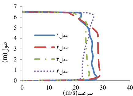
شکل ۵-۲۰- پروفایل سرعت محوری برای چهار مدل بر روی خط ۵ در سیکل ترکیبی
