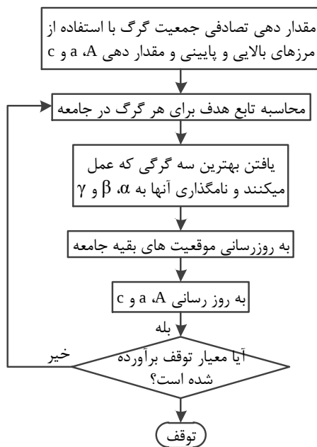
شکل (۱): فلوچارت الگوریتم GWO
