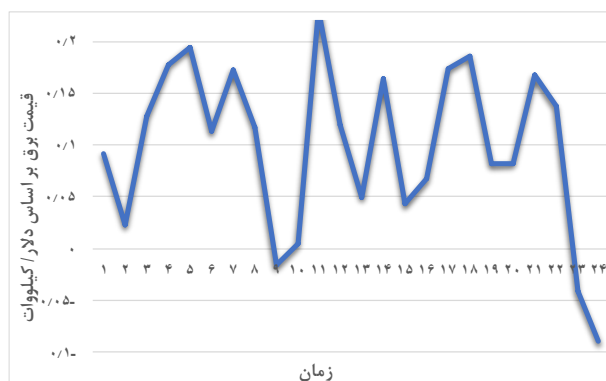
شکل (۴): تغییرات قیمت توان راکتیو در طی ۲۴ ساعت
