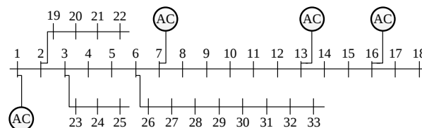
شکل (۲): سیستم ۳۳ باس IEEE
