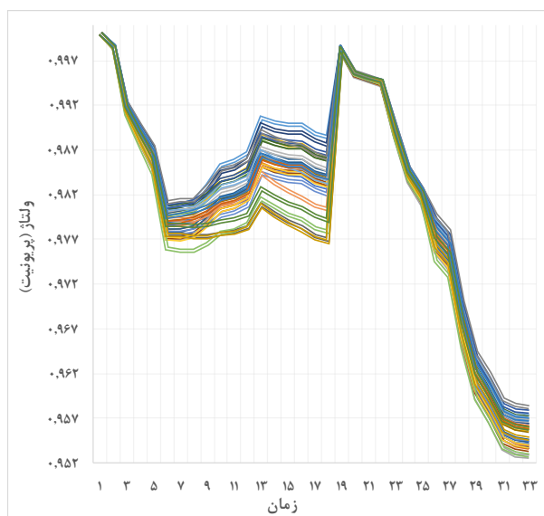
شکل (۳): انحرافات ولتاژ باس‌ها در سیستم ۳۳ باس IEEE
