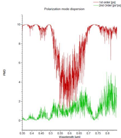
شکل ۶: پاشندگی مد پلاریزه (PMD) در طیف مرئی
