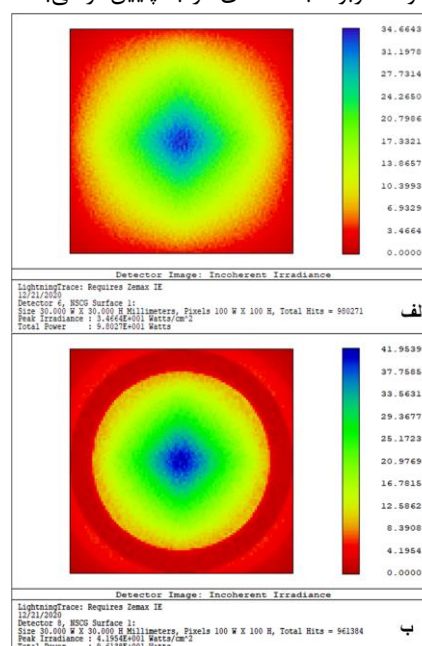
شکل (۷): نتیجه آشکارساز الف: قبل از لنز فرنل و ب: بعد از لنز فرنل
