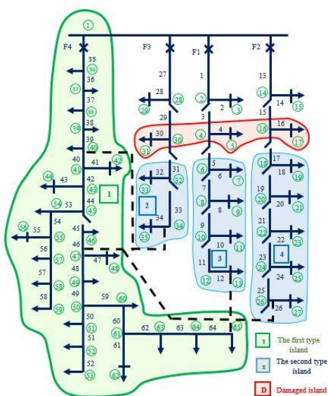
شکل ۵- توپولوژی جدید شبکه پس از احداث خطوط تایلین
