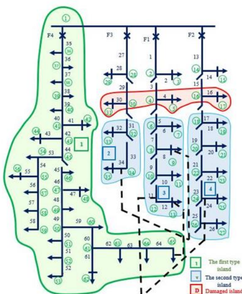
شکل ۱۲- آرایش جدید شبکه پس از احداث خطوط تای‌لاین در سناریو ۳
