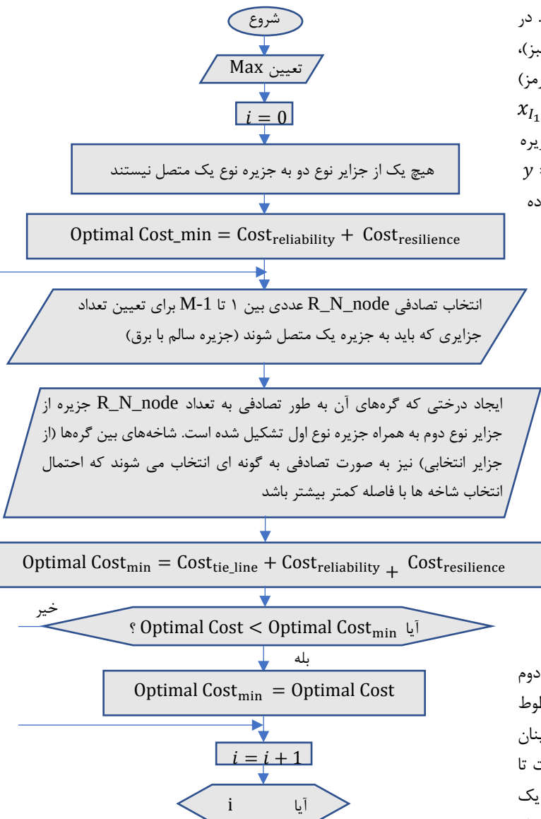
شکل ۳- فلوچارت الگوریتم پیشنهادی
