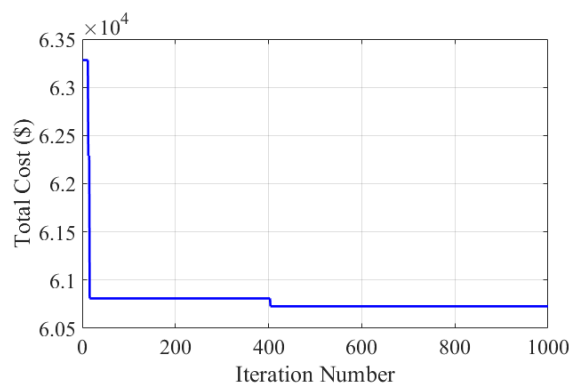
شکل ۱۰- منحنی همگرایی هزینه کل حاصل در سناریو ۲
