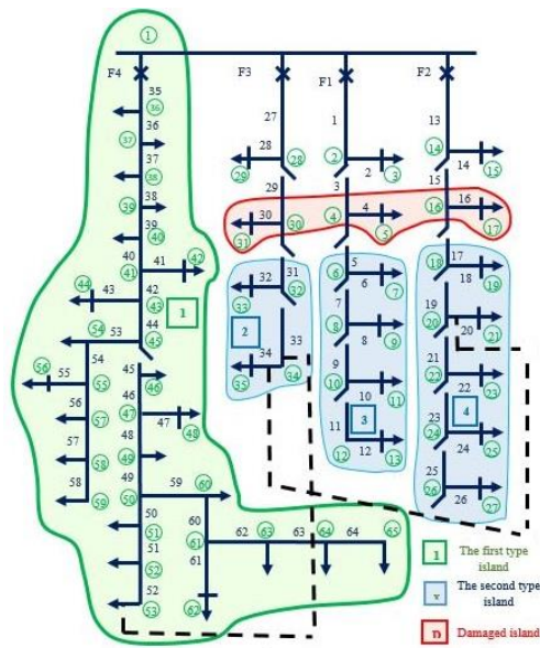
شکل ۹- آرایش جدید شبکه پس از احداث خطوط تایلین
