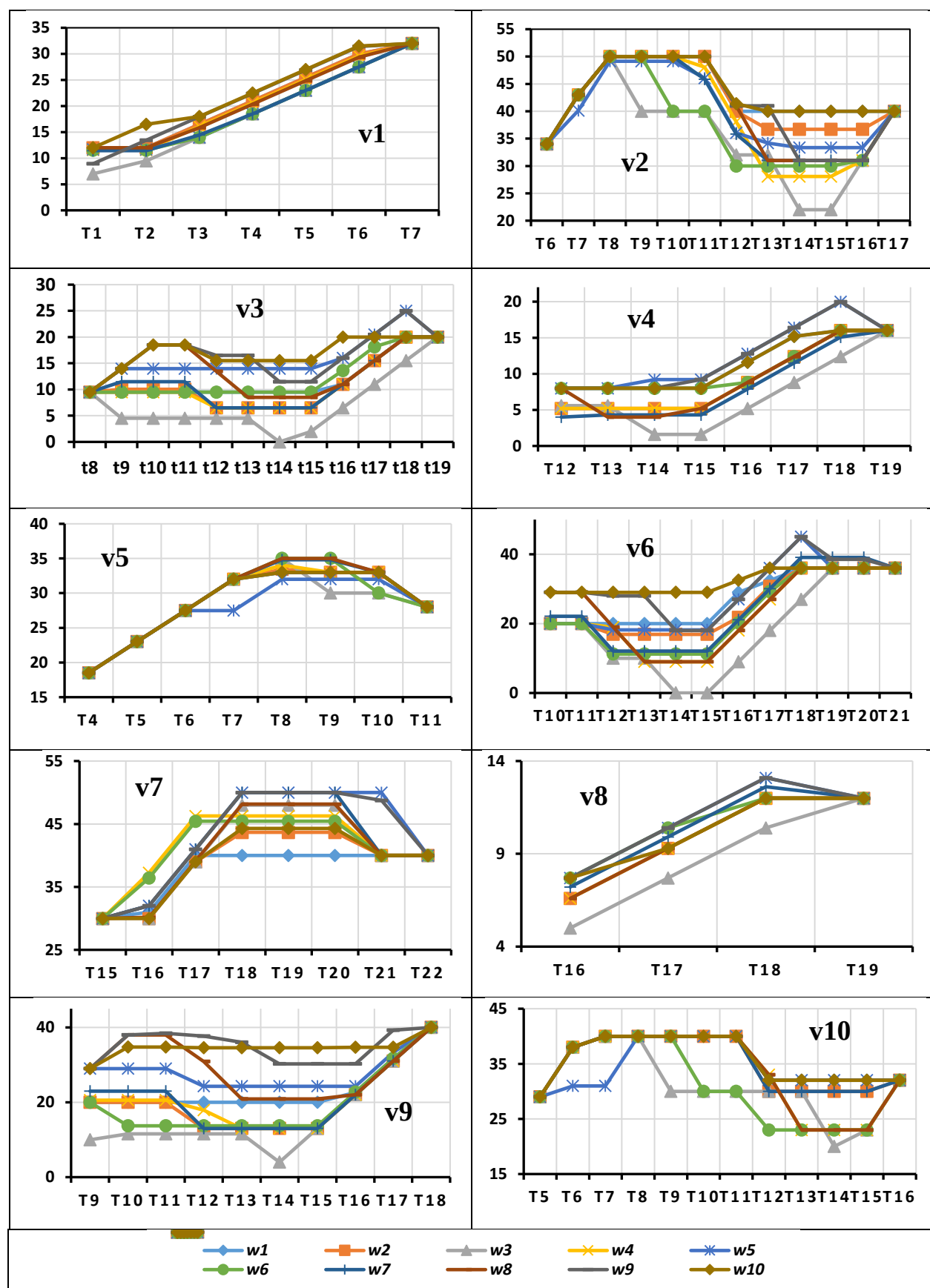
شکل (۸): سطح شارژ باتری خودروهای از دسته یک تا ده در تمامی سناریوها و دوره اتصال (محور افقی: زمان، محور عمودی: SOE (kWh))
