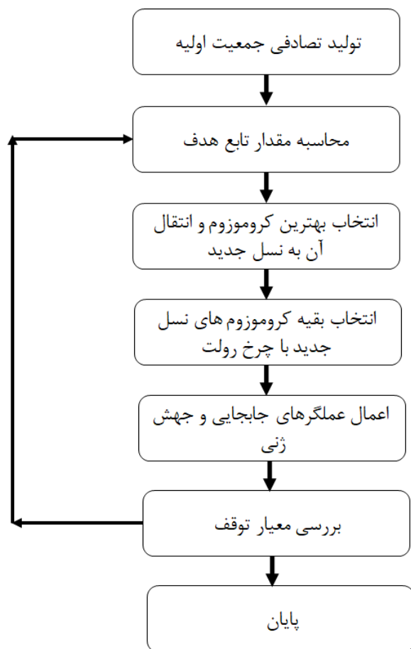
شکل ۴. فلوچارت الگوریتم پیشنهادی
