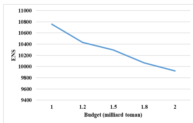
شکل ۱۲. روند بهبود شاخص انرژی تامین نشده (ENS) با افزایش بودجه اختصاص یافته
