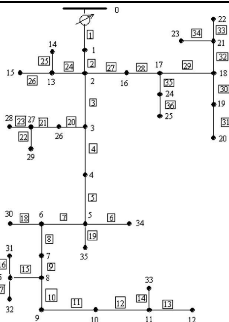
شکل ۵. شبکه تست ۳۷ با سه
