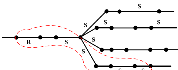
شکل ۳. نقض شرط حداکثر سکشن لایزهای تحت یک ریکلوز
