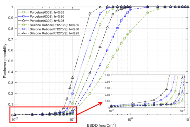
شکل (۲): احتمال تخلیه الکتریکی در مقره‌های سرامیکی و سیلیکونی در سطوح مختلف رطوبت و ESDD.
