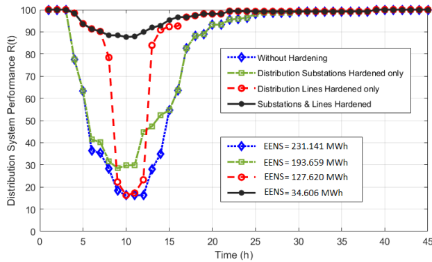
شکل (۶): نمودار تاب‌آوری سیستم توزیع در موارد مطالعاتی ۱ تا ۴.
