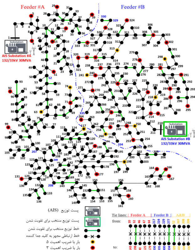
شکل (۷): نتایج برنامه‌ریزی تقویت همزمان خطوط و پست‌های توزیع.
