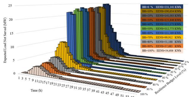
شکل (۹): تغییرات انرژی و بار تأمین نشده مورد انتظار در سطوح مختلف بودجه.
