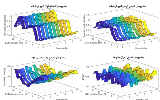
شکل (۵): سناریوهای تصادفی تغییرات بار و شرایط محیطی.
