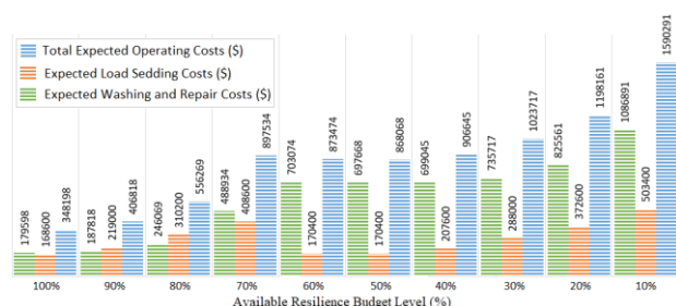
شکل (۸): هزینه‌های بهره‌برداری مورد انتظار در سطوح مختلف بودجه.
