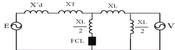
شکل (۹): سیستم دو باسه با خطای سه فاز در وسط خط با محدودساز
