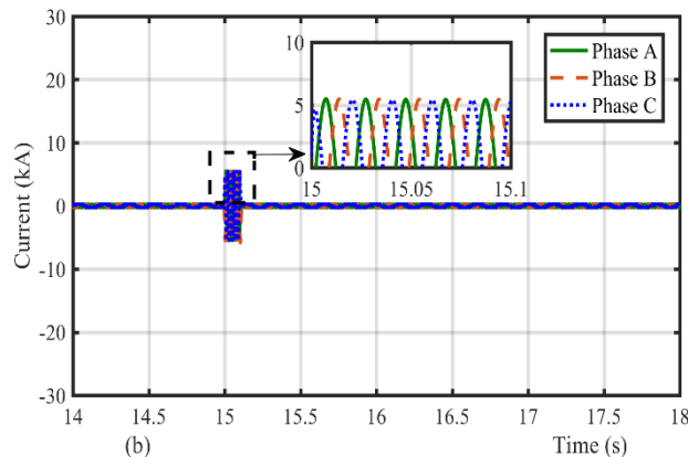
شکل (۱۵): جریان سه فاز فیدر ۱، الف) حالت اول ب) حالت دوم
