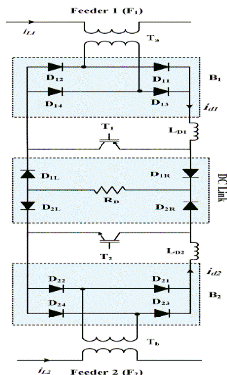
شکل (۲): ساختار محدود ساز بین خطی
