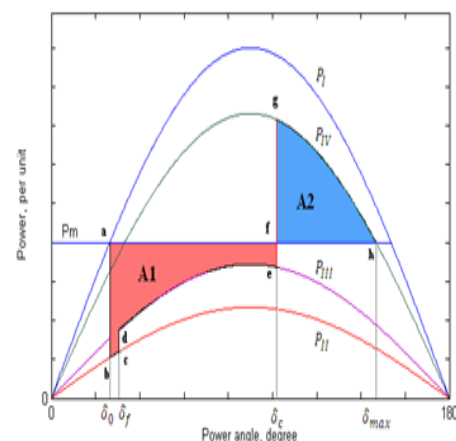
شکل (۱۱): منحنی توان-زاویه رتور پس از بکارگیری محدودساز
