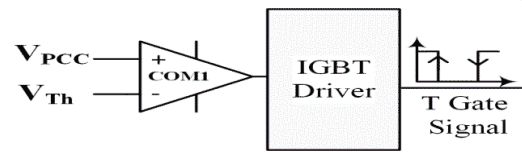
شکل (۹): سیستم کنترل محدود ساز بین خطی
