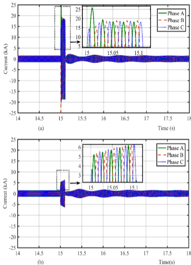
شکل (۱۴): جریانههای عبوری از پست ۲۳۰/۶۳ کیلوولت در شرایط اتصال کوتاه سه فاز به زمین در ابتدای فیدر شماره ۱، الف) حالت اول ب) حالت دوم
