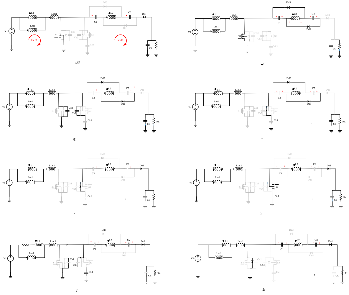
شکل (۵): حالت‌های عملکردی مبدل پیشنهادی
