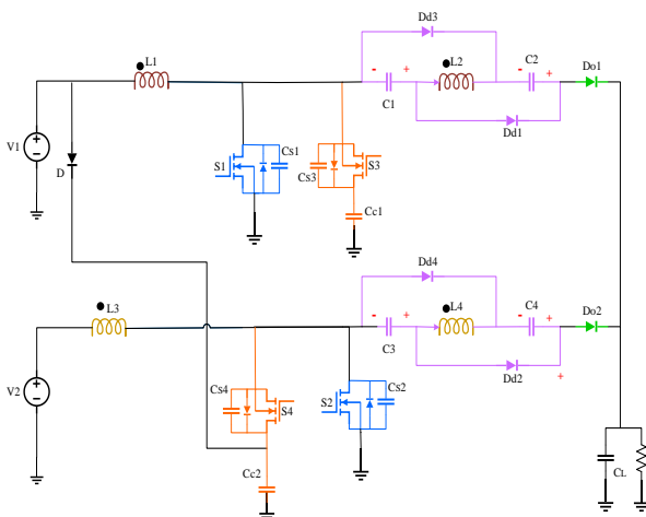
شکل (۳): ساختار مبدل پیشنهادی dc/dc چند ورودی غیر-ایزوله بهره بالا
