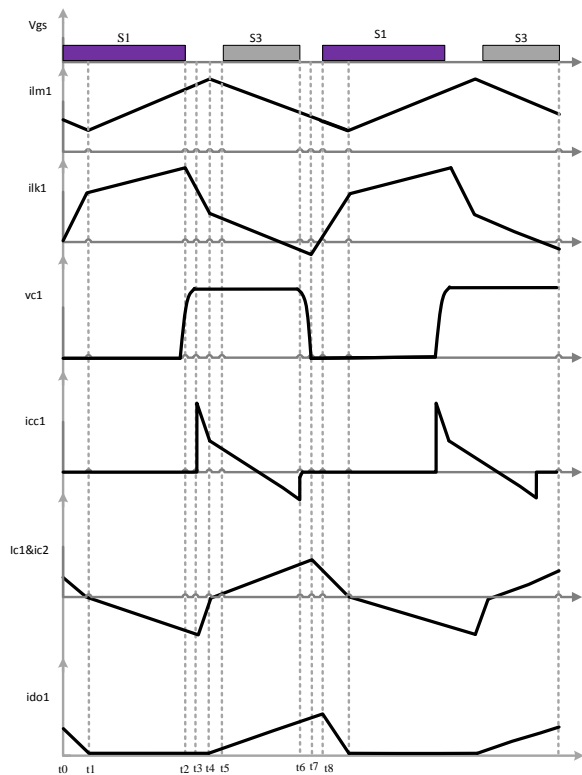
شکل (۴): شکل موج های اصلی مبدل پیشنهادی
