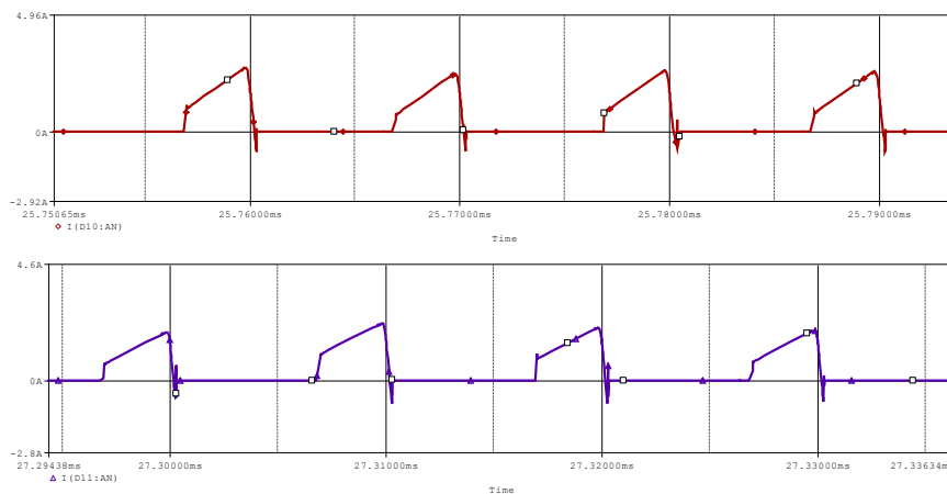
شکل (۱۲): موج جریان دیود خروجی در فاز بالا و پایین
