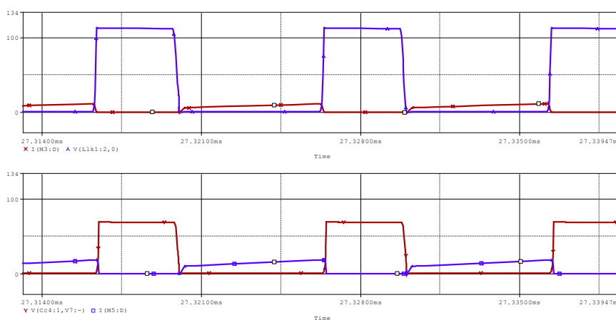
شکل (۱۳): وضعیت کلیدزنی نرم کلیدهای اصلی S_2 و S_1
