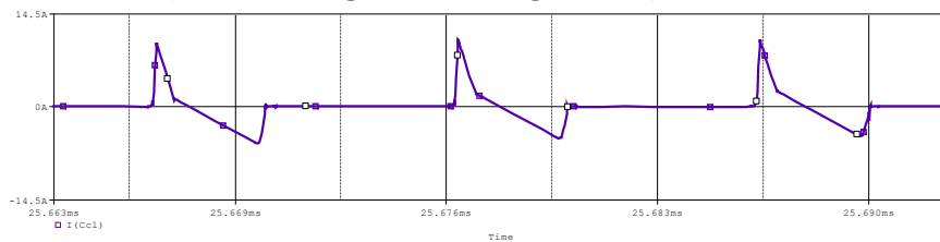
شکل (۹): جریان سلف نشتی و سلف مغناطیسی در فاز بالا و پایین
