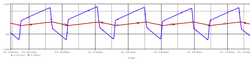
شکل (۹): جریان سلف نشتی و سلف مغناطیسی در فاز بالا و پایین
