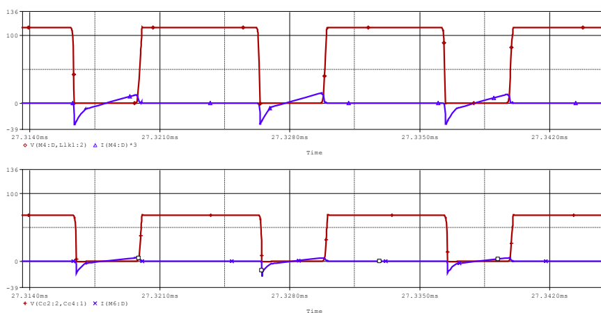
شکل (۱۴): وضعیت کلیدزنی نرم کلیدهای کمکی S_4 و S_3
