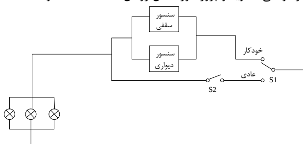
شکل (۱۰): مدار پیشنهادی برای سنسورها و لامپ‌ها
