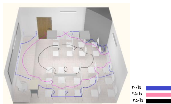
شکل (۳): شبیه‌سازی کلاس ۲۰۶ در نرم‌افزار دیالوکس
