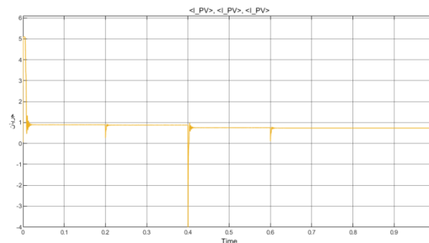
شکل ۱۲(پ) جریان ورودی روش PI
