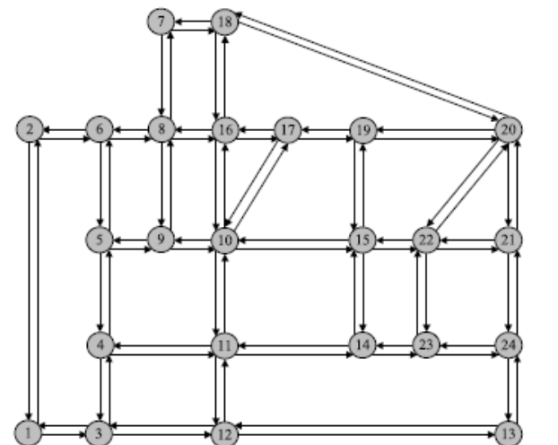
شکل (۴): شبکه ترافیک سوزان ۲۴ گره ای مورد مطالعه
