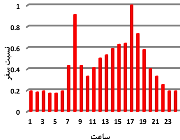
شکل (۶): پروفیل ساعتی جریان ترافیکی ماتریس O-D
