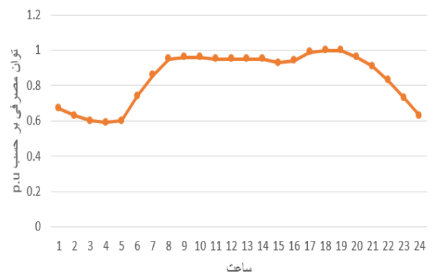
شکل (۵): نمودار بار روزانه مصرف کنندگان شبکه
