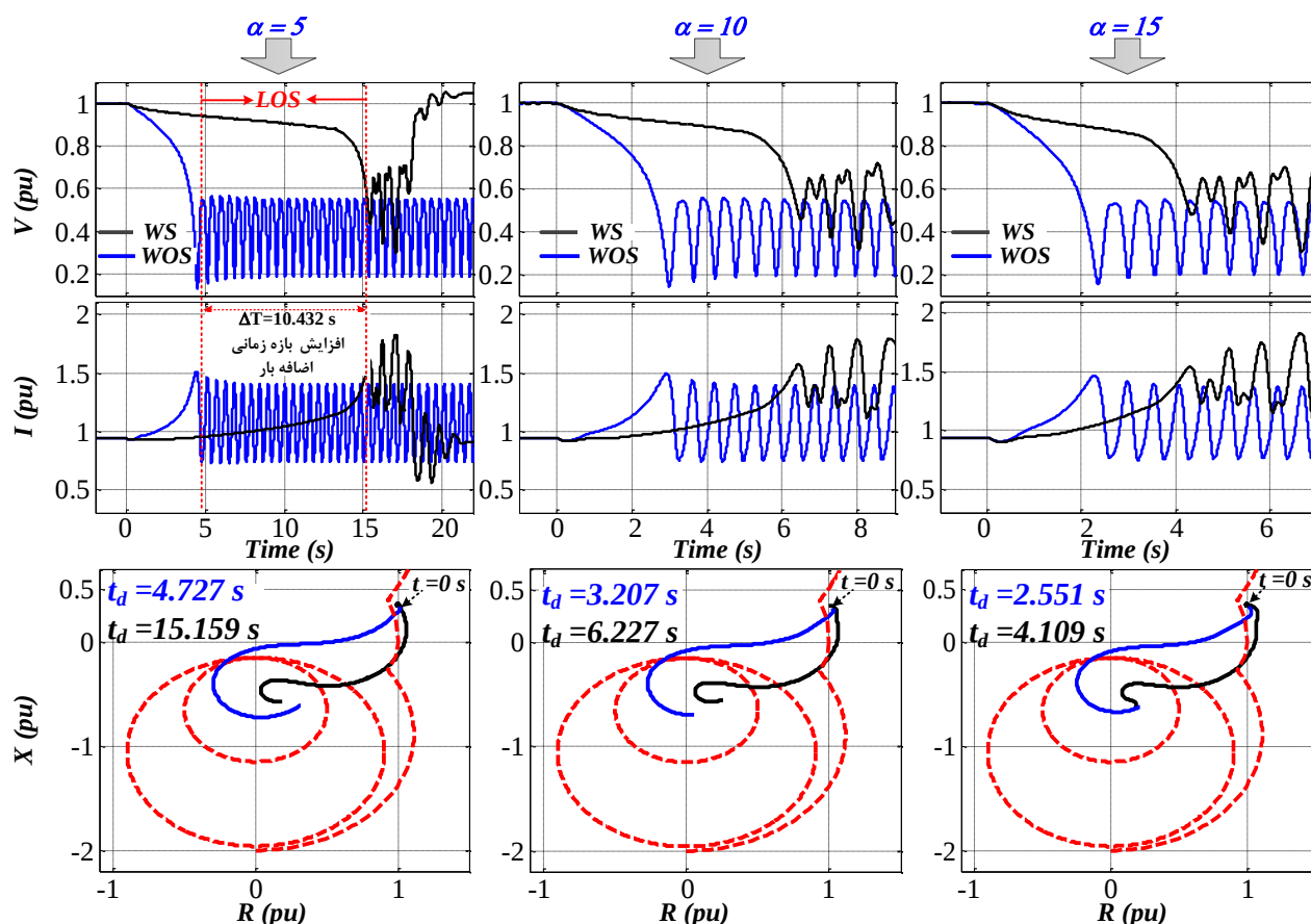
شکل (۹): تغییرات V و I به همراه عملکرد رله امپدانی در مواجهه با خطاهای PLOF در بارگذاری سنگین ژنراتور و در دو حالت: با حضور (منحنی‌های مشکی) و بدون حضور (منحنی‌های آبی) STATCOM.
