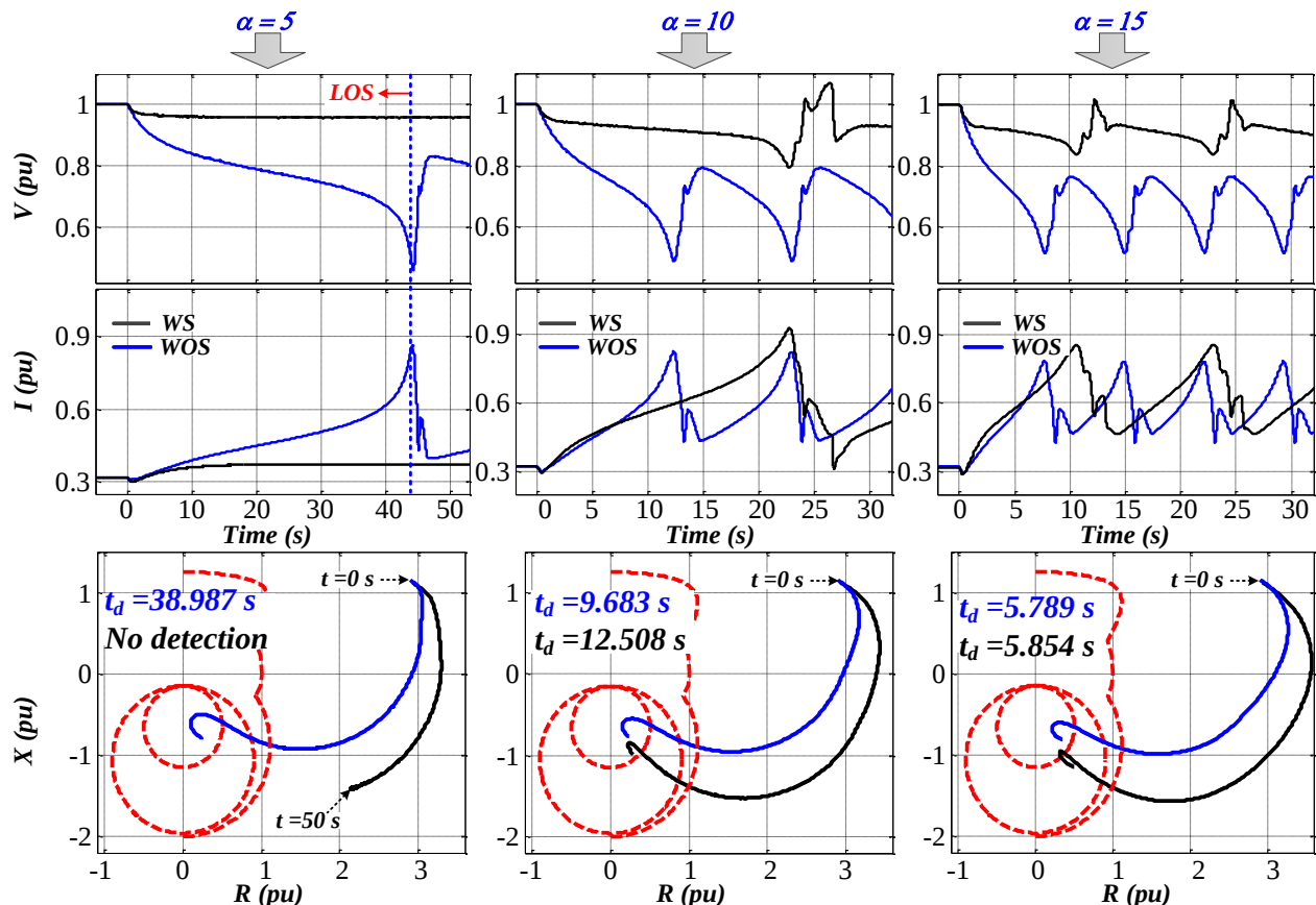
شکل (۱۰): تغییرات V و I به همراه عملکرد رله امپدانسی در مواجهه با خطاهای PLOF در بارگذاری سبک ژنراتور و در دو حالت: با حضور (منحنی‌های مشکی) و بدون حضور (منحنی‌های آبی) STATCOM.
