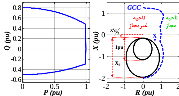
شکل (۴): منحنی GCC ژنراتور مورد مطالعه (چپ) و مشخصه عملکردی رله امپدانی در صفحه R-X
