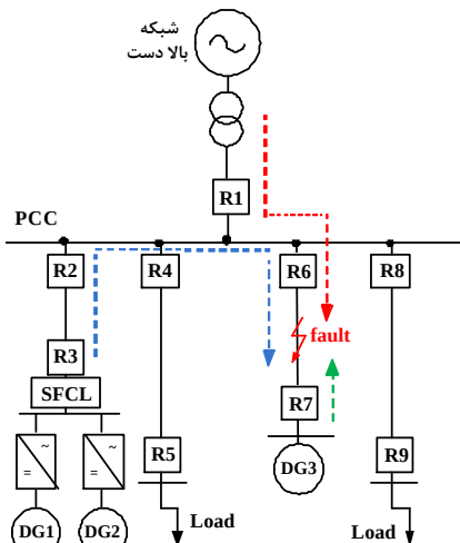
شکل (۹): ریز شبکه تحت ارزیابی در مطالعه مورد اول، حالت دوم.
