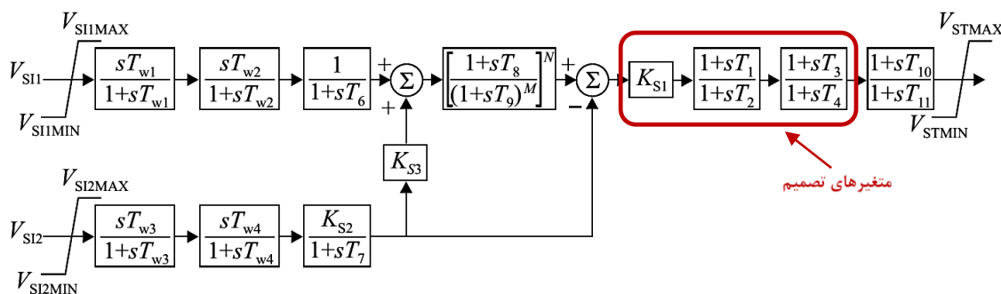
شکل (۵): متغیرهای تصمیم در بلوک دیگرام مدل استاندارد PSS
