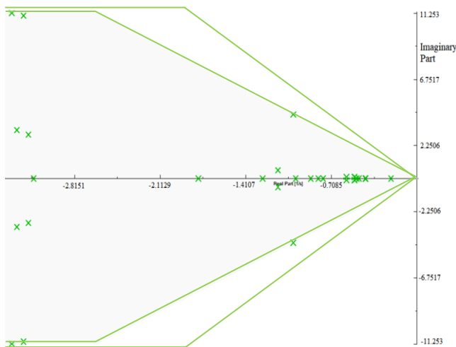
شکل (۱۰): وضعیت قرارگیری قطب‌های سیستم با پارامترهای بهینه شده PSS
