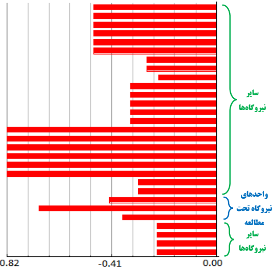
شکل (۱۲): ضرایب مشارکت نیروگاه‌های مؤثر بر نوسانات بین ناحیه‌ای وقتی فقط پارامترهای PSS یک واحد نیروگاه اصلاح شود.
